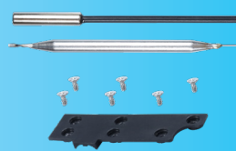
Kit de sortie arrière à distance pour capillaire, capteur de température et d'humidité
